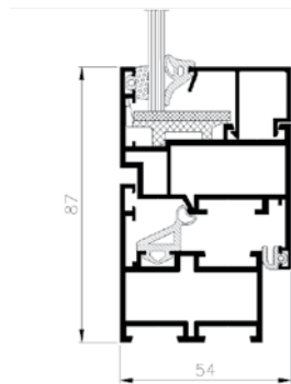
przekrój okna
